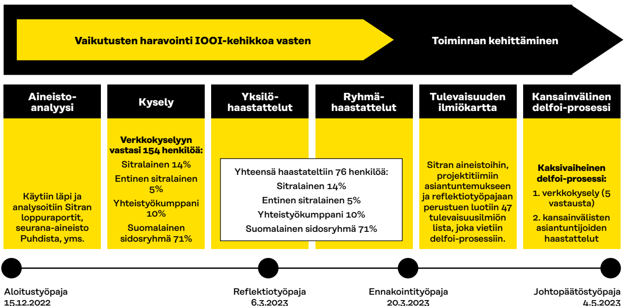
Kuva 2. Arvioinnin menetelmät.
